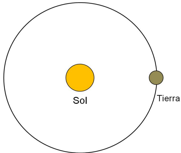
Figura 3.6: Órbita de la Tierra alrededor del Sol.
