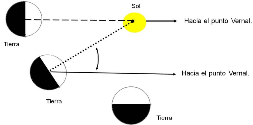
Figura 1.13: En esta figura se representan tres posiciones de la Tierra en su órbita. La línea a trazos denota la dirección entre un observador y el Sol. Para esa misma posición de la Tierra el Punto Vernal se ve en la misma dirección que el Sol. Las posiciones de la izquierda representan dos posiciones para dos días seguidos. La diferencia de posiciones está exagerada para ver que la Tierra gira un ángulo extra entre la culminación del Punto Vernal (línea continua) y la del Sol (línea punteada). Es decir, el Sol pasa por el meridiano del observador después que el Punto Vernal . Esto claramente ilustra que el día solar es mayor que el día sideral .
