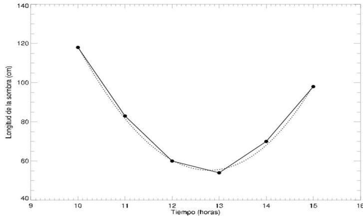
Figura 1.7: Gráfica de las extensiones de la sombra contra el tiempo. Se puede ver que la sombra llega a un valor mínimo y después vuelve a crecer. Con una línea punteada se indica la curva que se ajustó a los datos observados mediante un programa de ajuste de polinomios. La línea se puede dibujar a mano. En este caso, es conveniente hacer mediciones en intervalos de tiempo menores, por ejemplo, cada diez minutos para tener más precisión.
