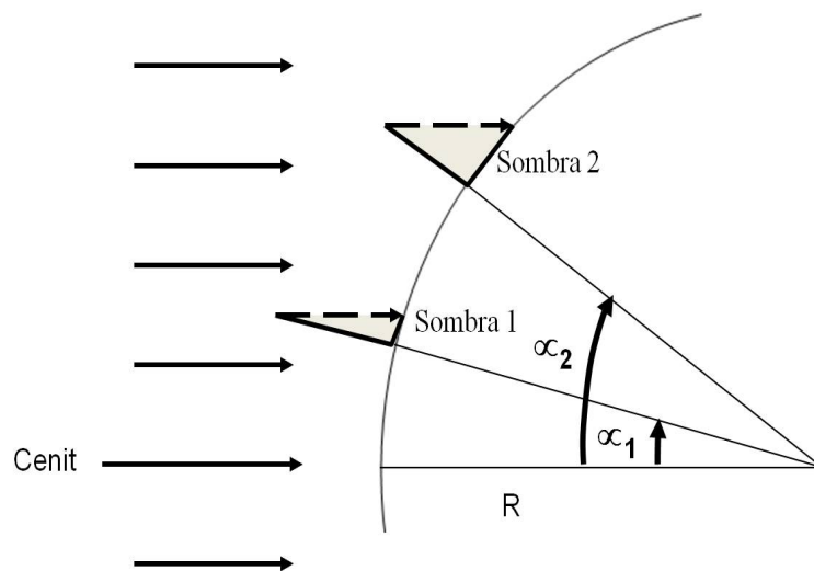
Figura 1.4: Representación de dos triángulos que se forman a partir de objetos verticales y sus sombras. Cada uno de estos triángulos tiene un triángulo semejante del centro de la Tierra hacia dichos lugares y hacia el lugar en el que no se produce sombra, es decir, a un lugar en el que el Sol está en el cenit durante su culminación .
