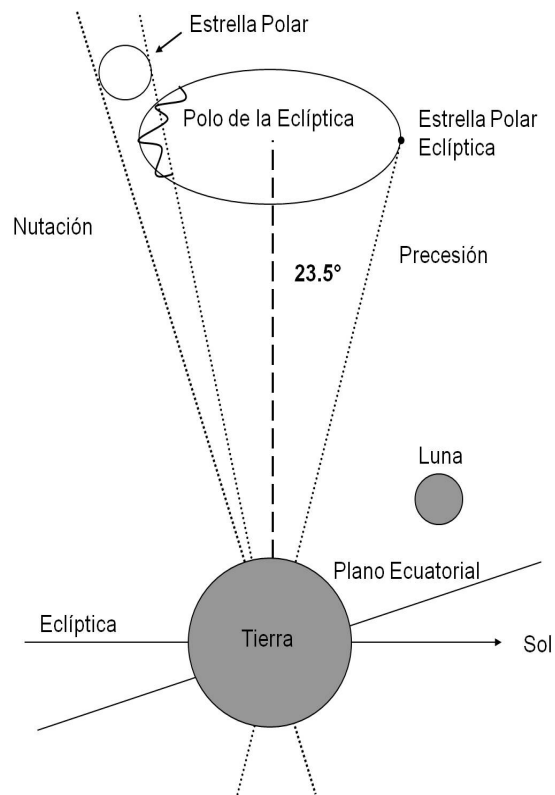
Figura 1.23: El movimiento de nutación se representa con la línea ondulada sobre la trayectoria del movimiento de precesión y de nutación . La línea horizontal representa a la eclíptica , la línea inclinada que cruza la Tierra representa al plano ecuatorial . La línea a trazos es perpendicular a la eclíptica y apunta hacia el polo de la eclíptica . La línea punteada del lado derecho representa la dirección a la que actualmente apunta el Eje Polar . La elipse (vista así por la proyección) representa la trayectoria del Eje Polar debido a la precesión a lo largo de 26000 años. Las líneas punteadas de la izquierda representan las posiciones extremas del eje polar debido al movimiento de nutación .
