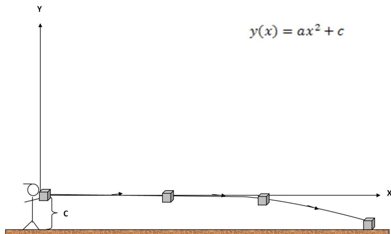
Figura 4.2: Trayectoria de un objeto lanzado a una altura C sobre el suelo, en dirección paralela a éste.
