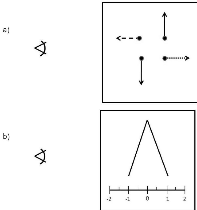
Figura 2.3: a) Representación de un sistema con cuatro partículas. Las flechas son vectores que representan las velocidades de las partículas, la longitud indica la magnitud de la velocidad (todas tienen la misma magnitud) y la dirección indica la dirección en la que se mueve la partícula. Para hacer más esquemático el dibujo todas las flechas apuntan hacia afuera, esto se hizo así para que se pueda visualizar más claramente que las partículas se mueven en distintas direcciones. b) Representación del número de partículas que ve el observador en cada dirección hacia él ve solo una, la cual está en " - 1" alejándose de él también ve solo una (que está en 1) y en direcciones transversales ve dos partículas. Debido a la dirección en la que se mueven estas dos partículas no producen desplazamiento Doppler y por eso están en "0".
