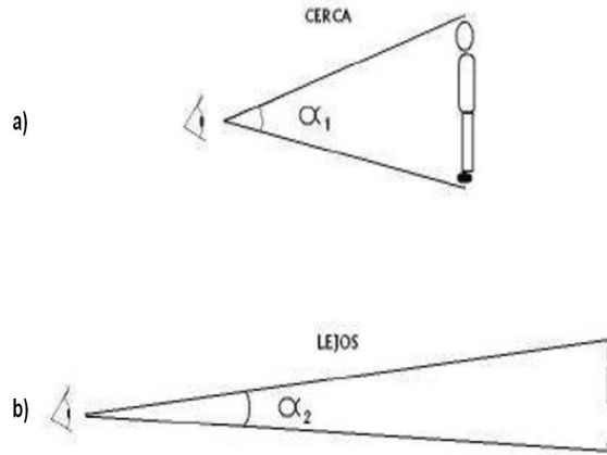
Figura A.5: a) Ángulo subtendido por una persona estando cerca del observador. b) Ángulo subtendido por la persona pero ahora cuando está lejos del observador. Se puede ver que el ángulo subtendido es mayor cuando la persona está más cerca. A medida que se vaya alejando del observador el ángulo que subtiende será menor.
