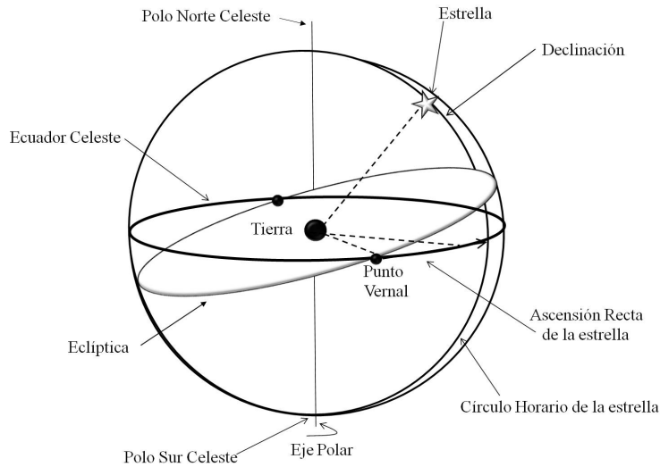
Figura 1.20: En esta figura se representa a la Tierra en el centro de la esfera Celeste. La línea vertical es la extensión del eje polar , la línea gruesa denota al Ecuador Celeste, el cual es perpendicular al eje polar . Sobre el Ecuador Celeste hay otra referencia que es el Punto Vernal . A partir del Punto Vernal se mide la ascensión recta como lo indica la flecha sobre el Ecuador Celeste. La declinación se mide a lo largo del círculo horario , desde el Ecuador hasta la estrella.
