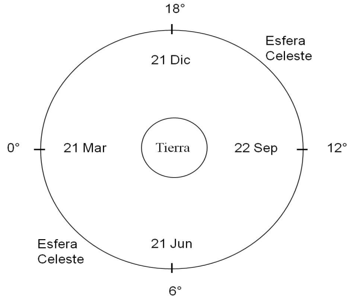
Figura 1.11: Representación de cuatro ascensiones rectas del Sol en la esfera Celeste. Cada una de las posiciones del Sol corresponde a un cambio de estación del año. Si el Sol está a 0^\circ entonces durante la noche vemos las estrellas que están entre 6^\circ y 18^\circ grados de ascensión recta . Si el Sol está a 12^\circ entonces durante la noche vemos las estrellas cuya ascensión recta es mayor a 18^\circ grados y menor a 6^\circ .
