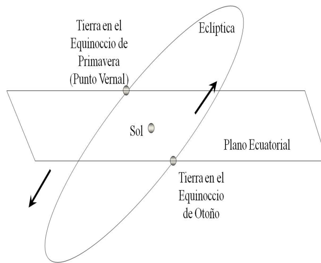
Figura 1.19: El Ecuador de la Tierra no es paralelo al plano de la eclíptica (en el que la Tierra gira alrededor del Sol). El ángulo que se forma entre el plano ecuatorial y el plano de la eclíptica es de 23.5^\circ . En esta figura exageramos la inclinación de la eclíptica para hacer más esquemática la diferencia entre el plano ecuatorial y las posiciones de la Tierra en su órbita. El eje de rotación es perpendicular al Plano Ecuatorial entonces cuando la Tierra está en el lado derecho le da más luz del Sol al hemisferio Sur y cuando está del lado izquierdo le da más luz al hemisferio Norte. En esta figura tenemos en el centro al Sol, visto desde la Tierra el Sol se ve en el Sur cuando la Tierra está por encima del plano ecuatorial , lo cual ocurre después del equinoccio de otoño , hasta el equinoccio de primavera . Ese trayecto de su órbita está en el lado derecho de la Figura 1.17
