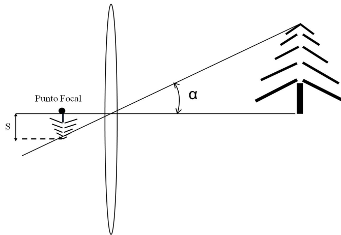
Figura 2.2: Imagen de un árbol en una placa fotográfica después de pasar la luz procedente del árbol por una lente. En la placa el árbol tiene un tamaño s mientras que el ángulo que subtende visto desde la lente es \alpha .
