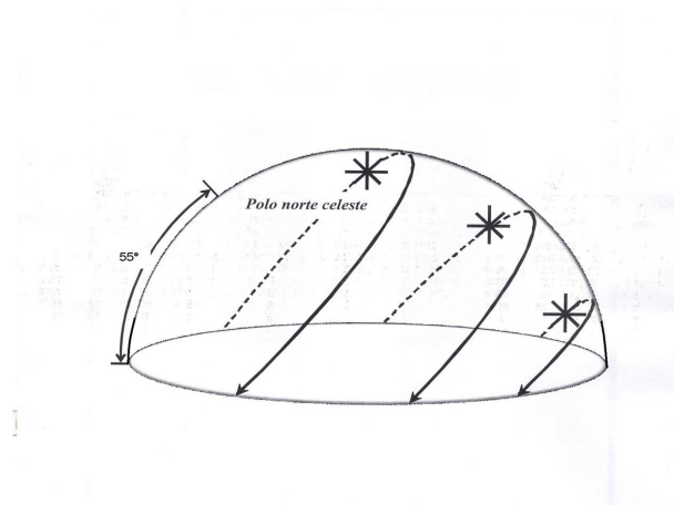
Figura 1.16: Trayectorias de las estrellas como las ve un observador en la ciudad de Moscú a 55^\circ de latitud Norte . Para un observador en esta latitud las trayectorias son muy inclinadas respecto del plano horizontal del observador.
