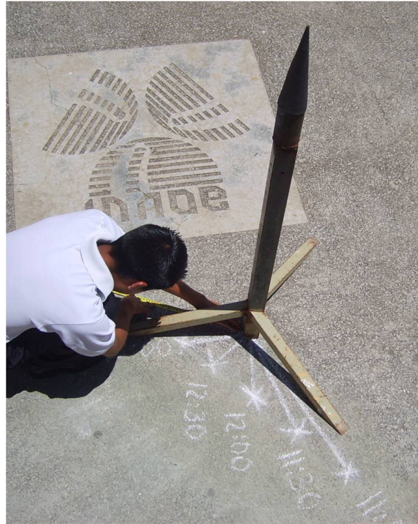
Figura 1.6: Trazos de las sombras del tripié en el suelo para varios tiempos. En el extremo de la sombra se trazó una cruz para denotar la longitud de la sombra en cada tiempo. Los tiempos están anotados junto a la cada línea.
