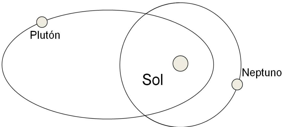
Figura 3.7: En esta figura se representa la órbita de Neptuno (línea punteada) que es casi circular. La elipse representa la órbita de Plutón (línea a trazos).
